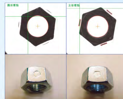
360° 外部檢測 360° External Inspection
