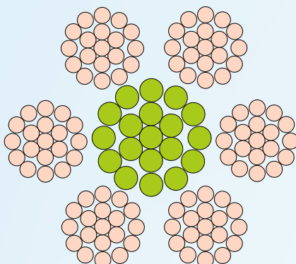
K6 x 19+IWS(7 x 19)
