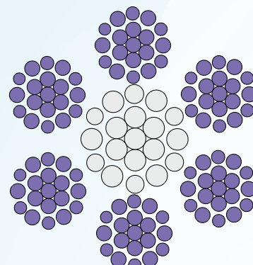
K6 x 19W+IWS(7 x 19)
