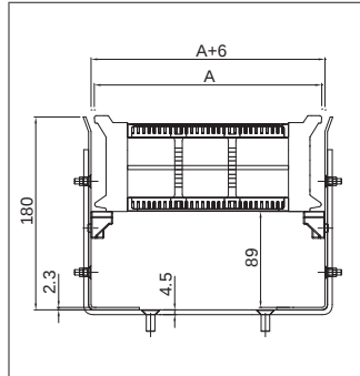
C-zone
