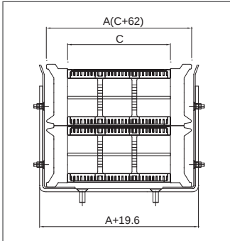
A-zone
