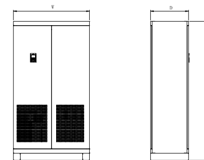
e) GK800-4T560~GK800-4T630
