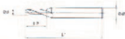
TEK AĞIZLI HSS FREZE UÇLARI
