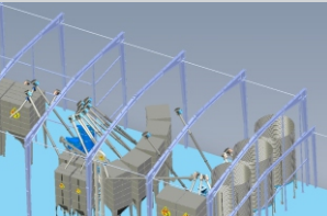
Mešaone stočne hrane
