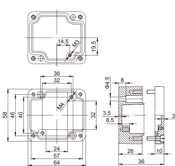
型號：DA111 重量：0.16kg 規格：58x64x36mm Model：DA111 Weight：0.16kg Size：58x64x36mm
