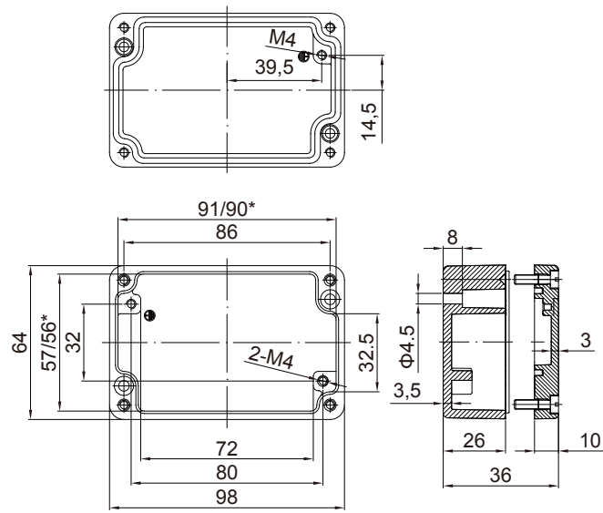
型號：DA121 重量：0.23kg 規格：64x98x36mm Model：DA121 Weight：0.23kg Size：64x98x36mm
