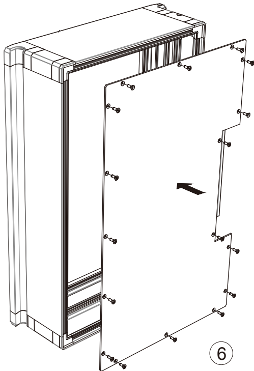
5. 安裝後門板 Install the rear panel.
