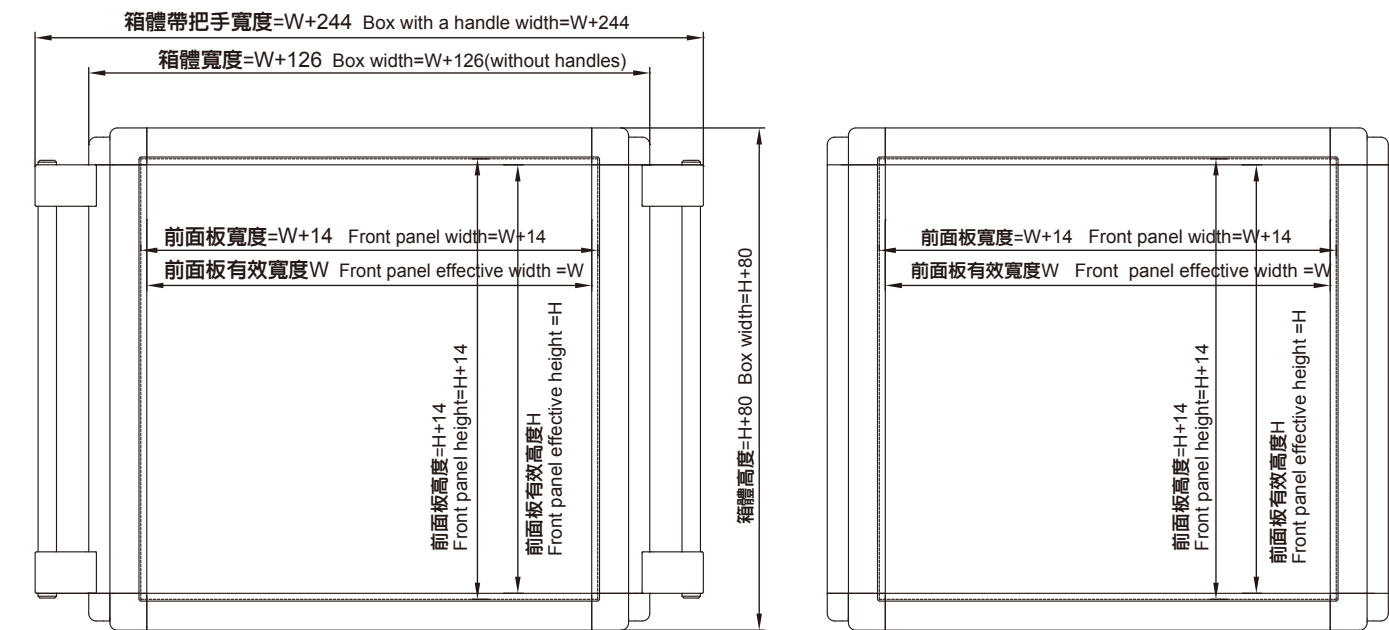
DST200/DST130 箱體尺寸 DST200/DST130 Box size
