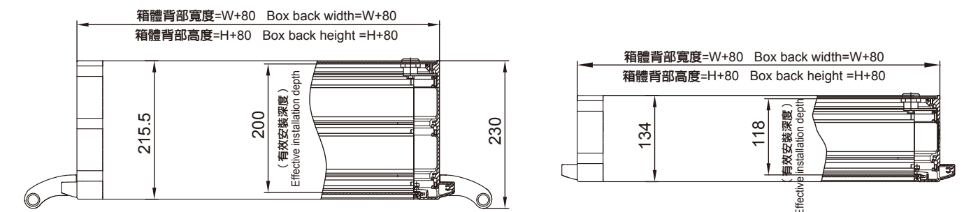
DST200/DST130 箱體尺寸 DST200/DST130 Box size
