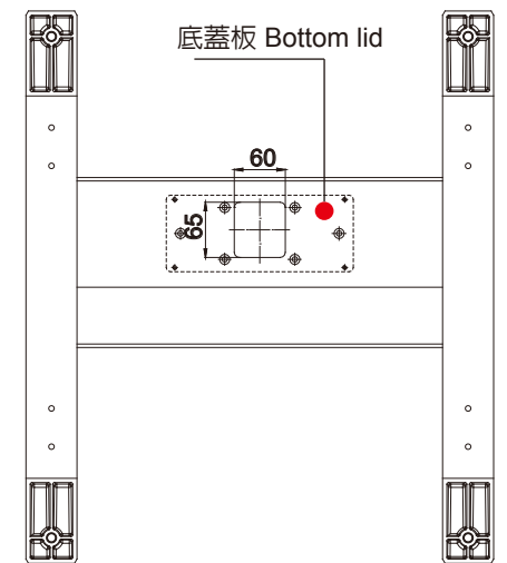
立柱底部 B向出線口 The outlet in the middle bottom (Direction B)
