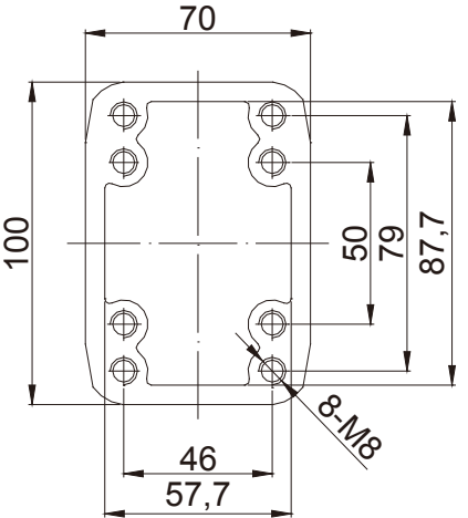
70100鋁管 70100 Aluminum tube
