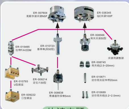
快速夾頭
