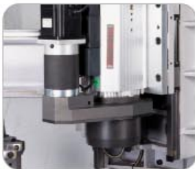
▲ C axis C軸 (四軸聯動)
