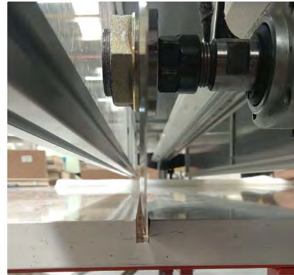
Sheet & Blanket Cutting Machine / Tafel- und Deckblattschneidmaschine
