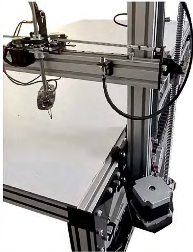
CNC Shaped Hot Wire Cutting Machine / CNC-geformte Heißdrahtschneidemaschine
