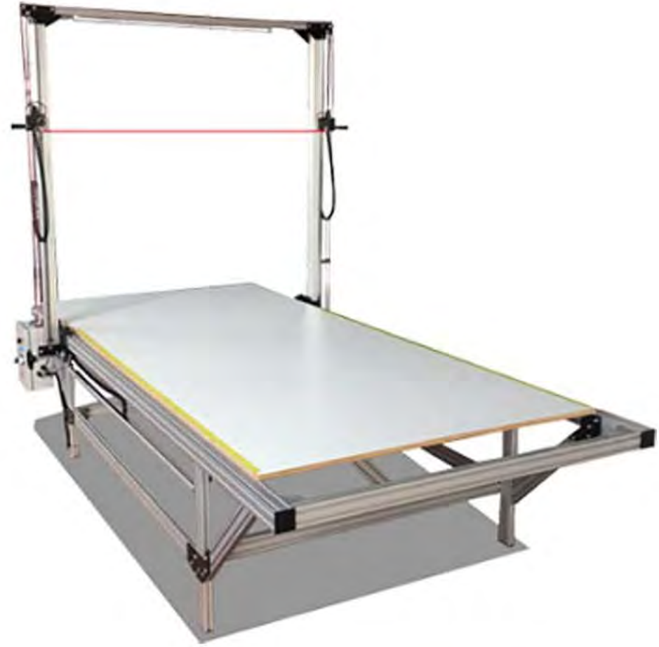
Manual Styrofoam Guillotine 2-Way Slitting / Manuelle Styropor-Guillotine 2-Richtungs-Schneiden
