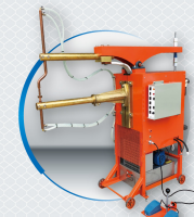
Pneumatic Stationary Type / 空壓立式
