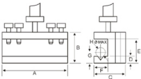
VEE Groove Holder
